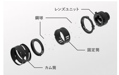
ダイナミックローリングカム機構
